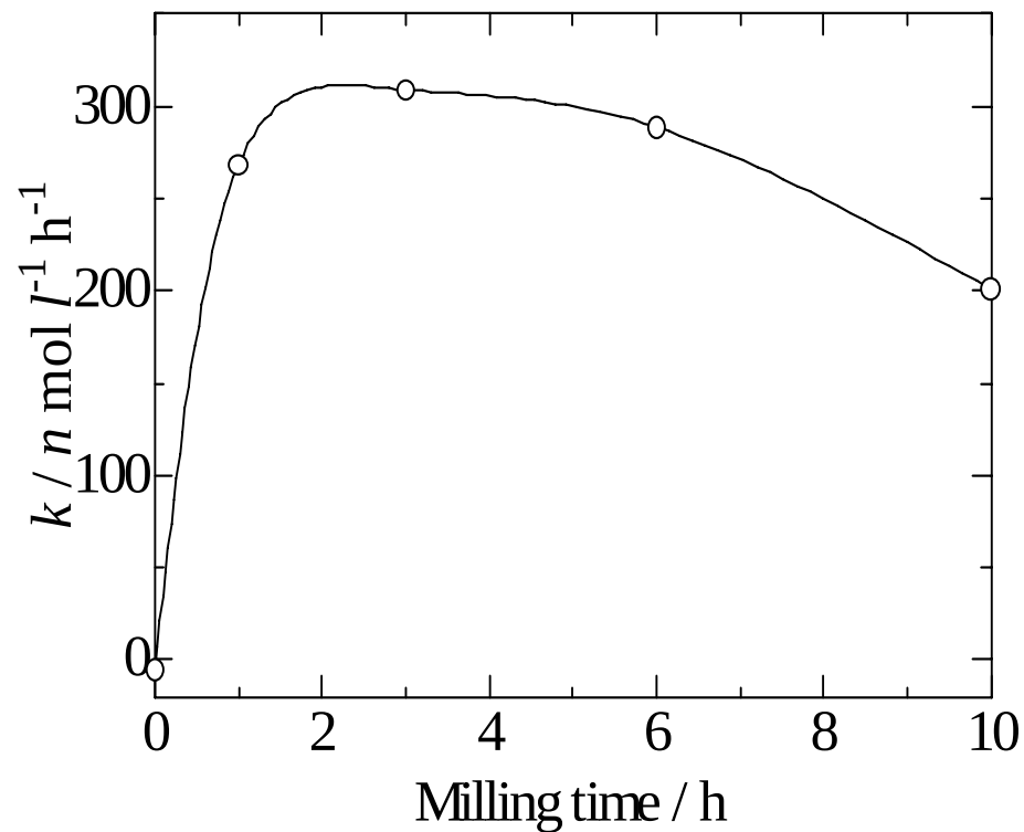
複合光触媒薄膜ボールによる MB分解速度係数
