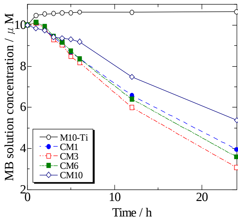
複合光触媒薄膜ボールによるMB分解
